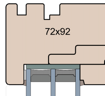
Nadproże
