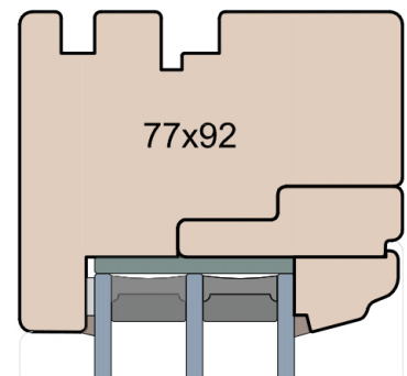
Nadproże
