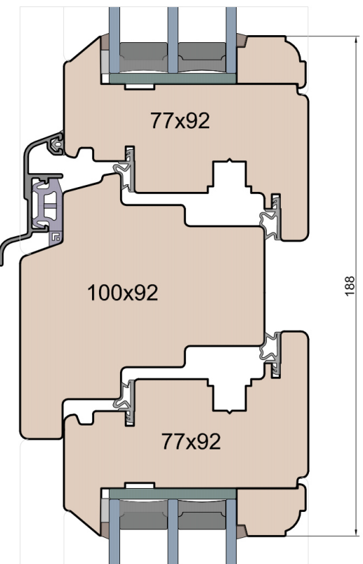
Rygiel
