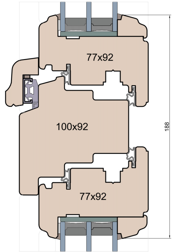
Rygiel
