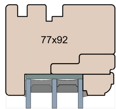
Nadproże
