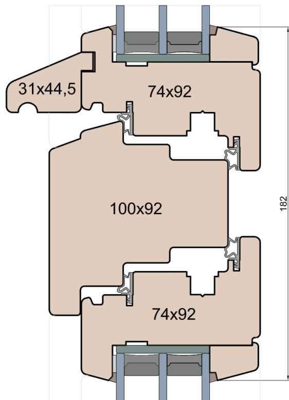
Rygiel
