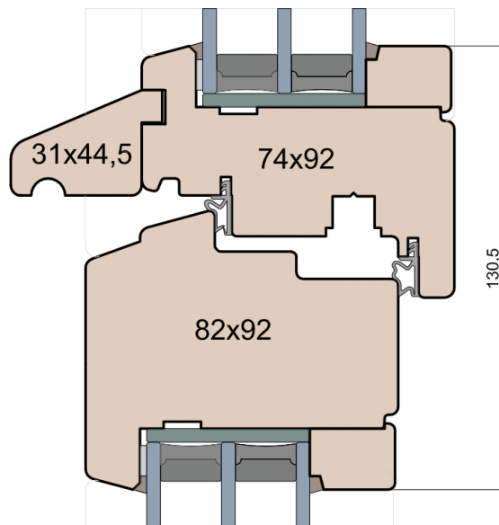
Nadproże
